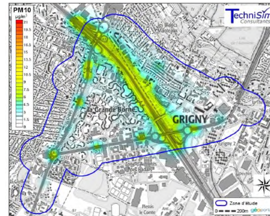
Figure 171 – Horizon 2019 actuel – concentration (µg/m³) moyenne annuelle PM10
