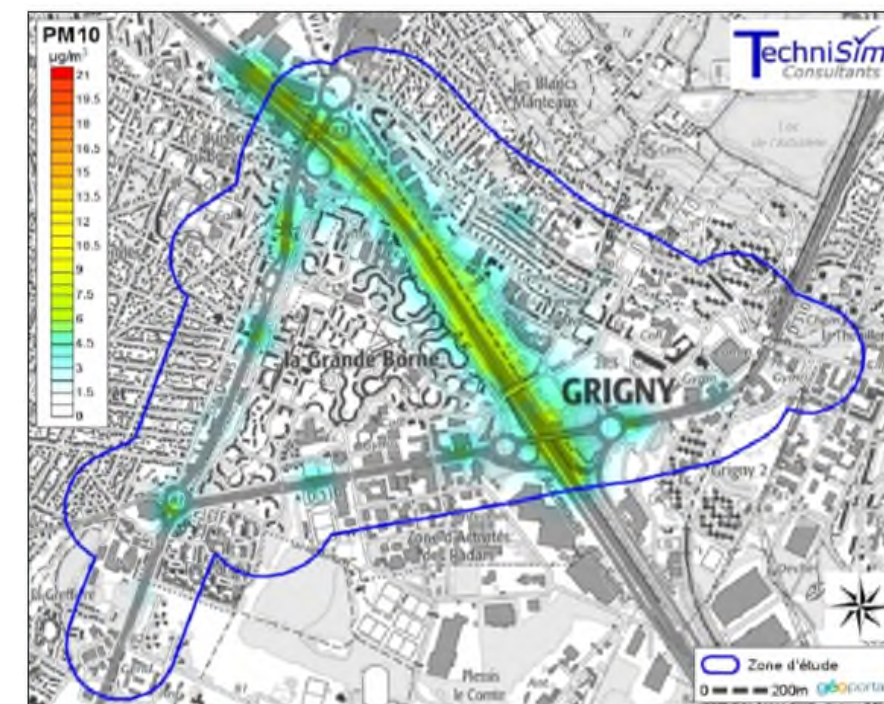
Figure 172 – Horizon 2025 fil de l'eau – concentration (µg/m³) moyenne annuelle PM10
