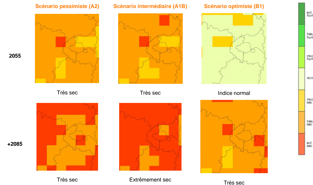
Figure 184 – Indicateurs de sécheresse/d'humidité des sols, saison estivale (Source : DRIAS, 2020)
