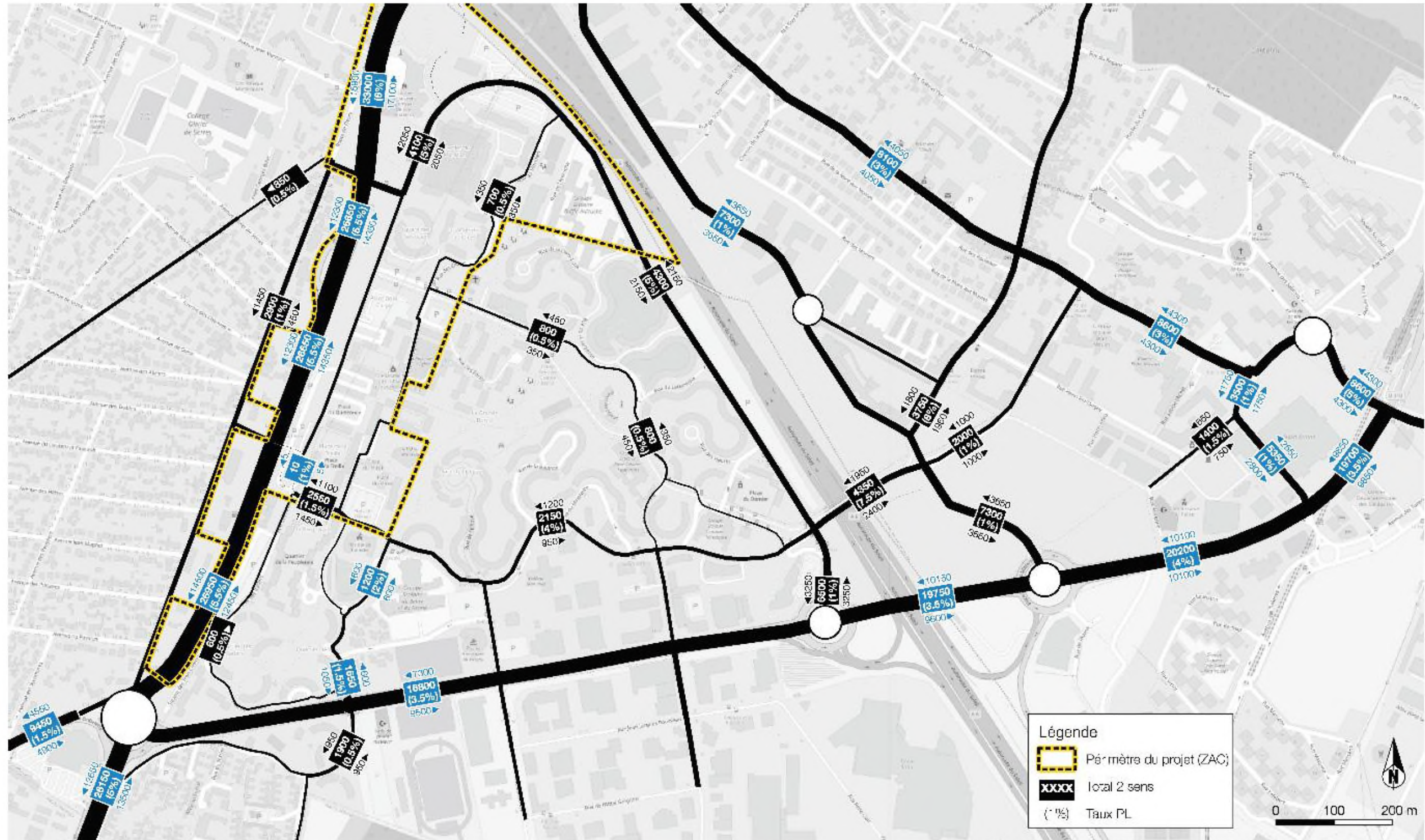
Figure 144 – Demande de trafic journalier lié au projet – Projection à l’horizon 2025, Trafic Journalier Moyen Annuel
